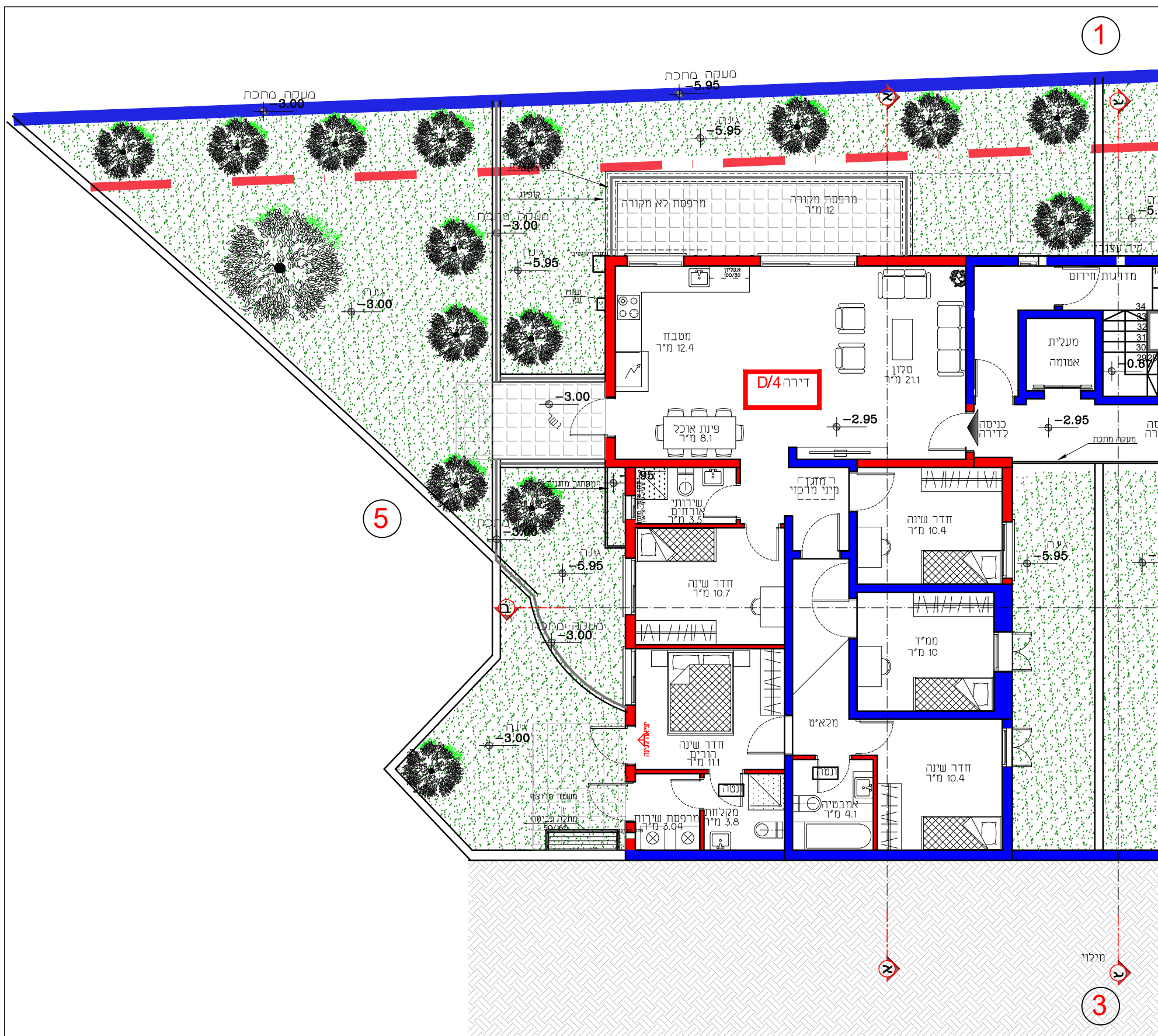
D בניין תכנית מפלס -2.95 קנ"מ 1:100
