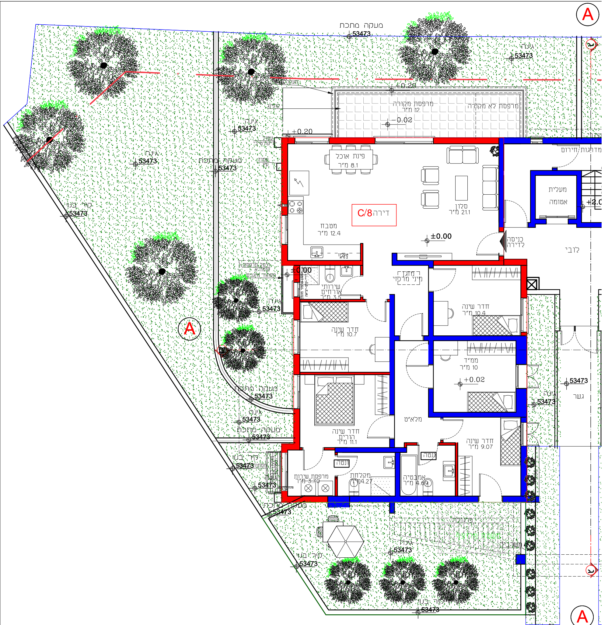
בניין C תכנית מפלס ±0.00 קנ"מ 1:100
