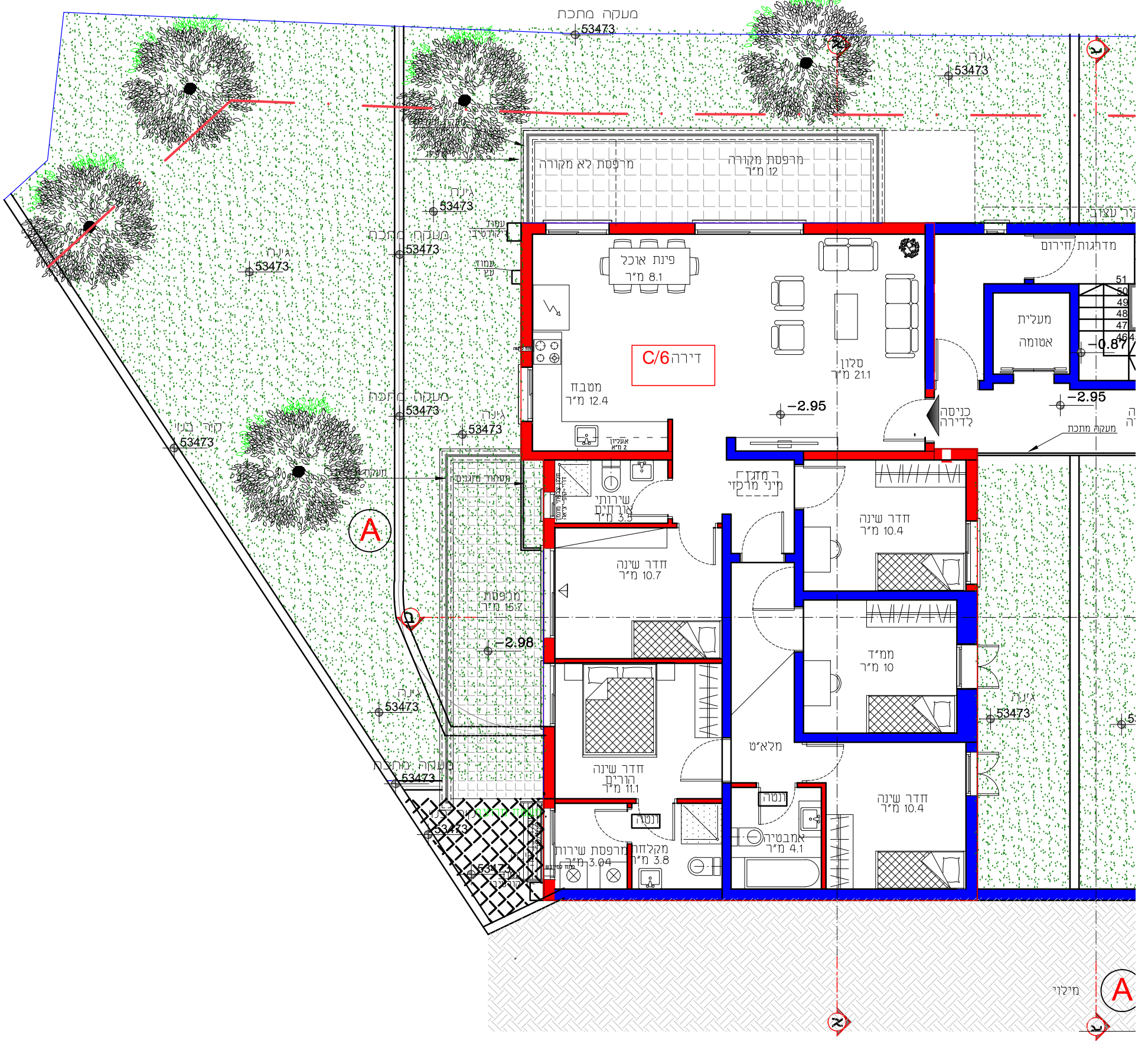
בניין C תכנית מפלס -2.95 קנ"מ 1:100
