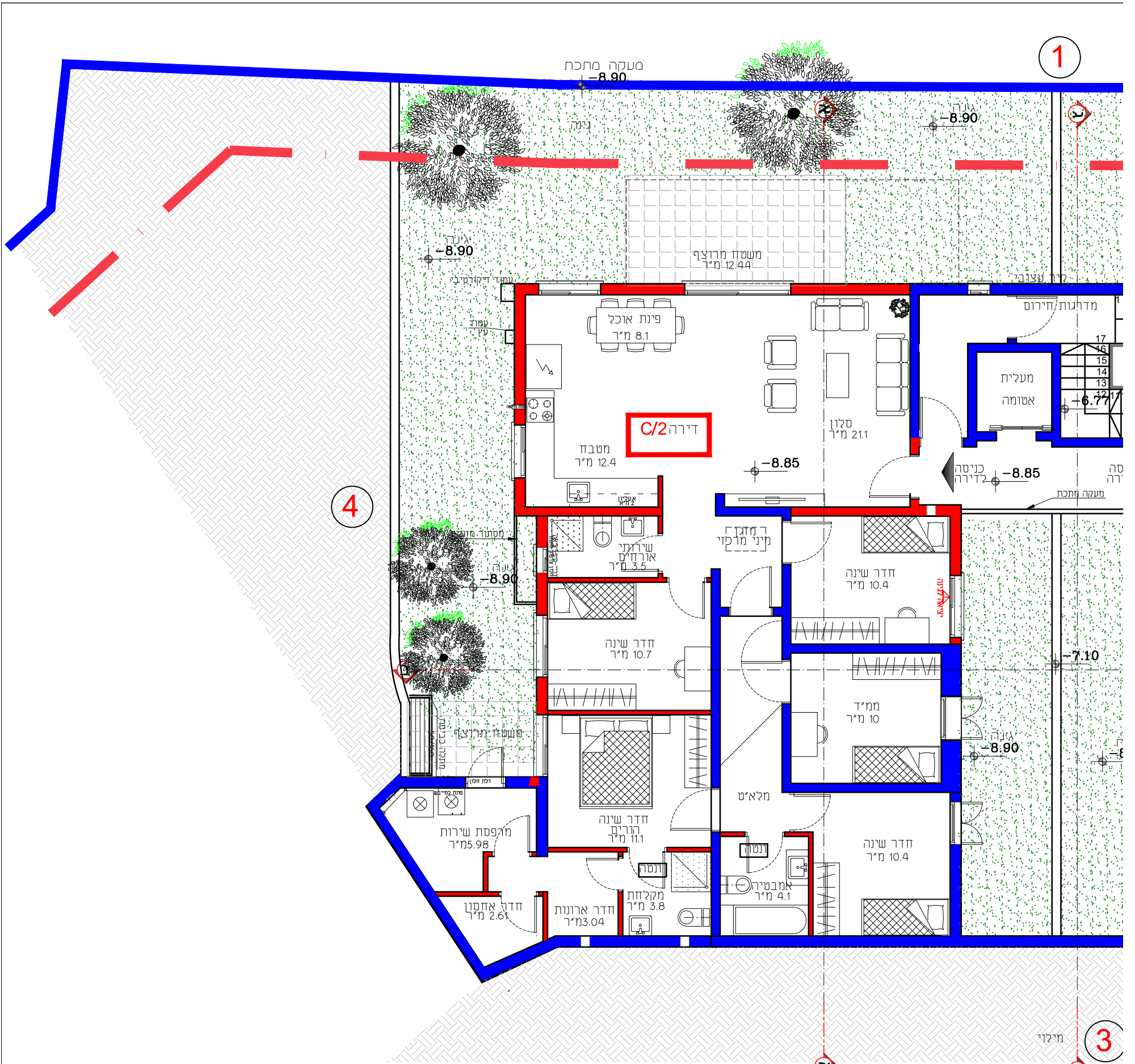
בניין C תכנית מפלס -8.85 קנ"מ 1:100
