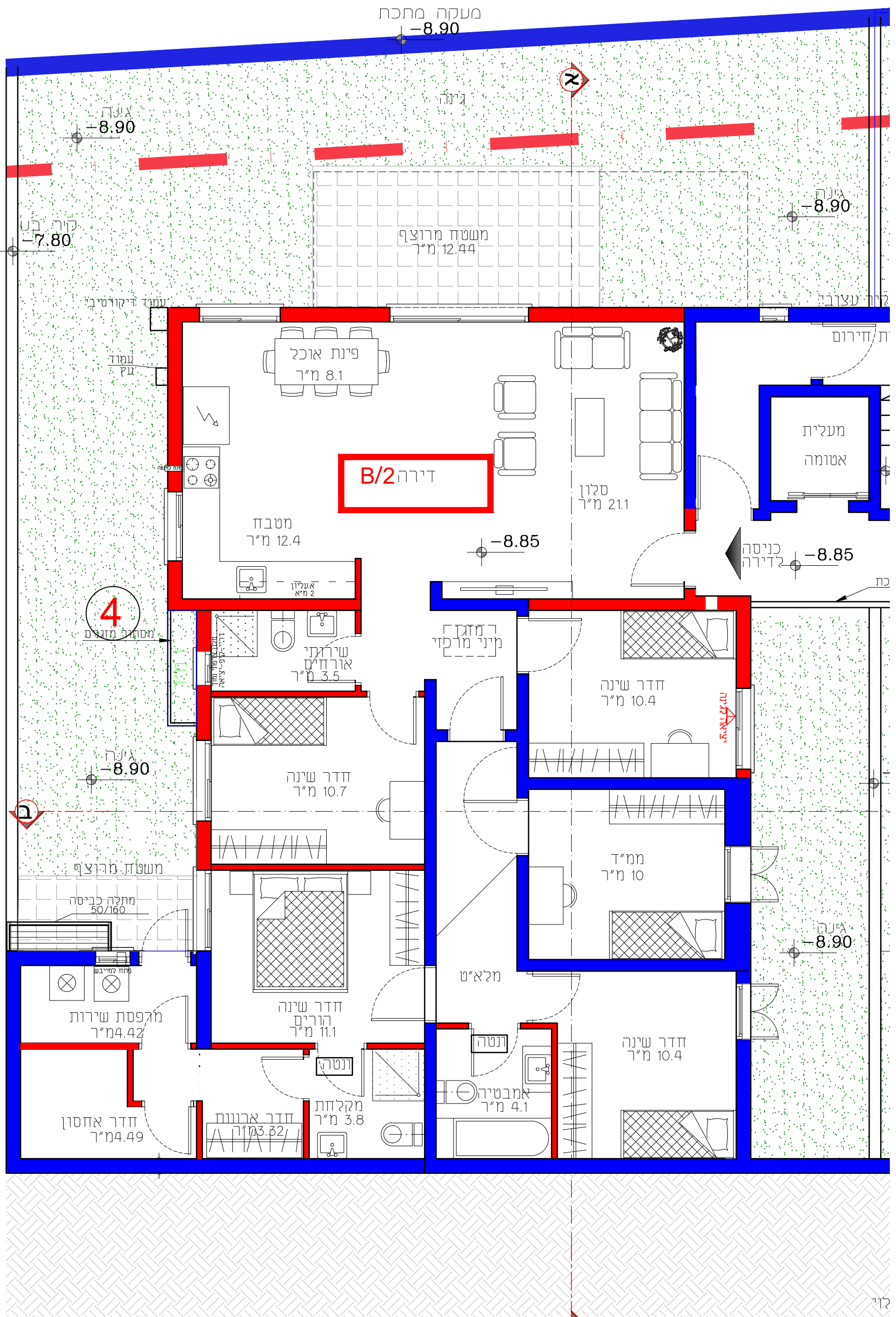
B בניין תכנית מפלס -8.85 קנ"מ 1:100
