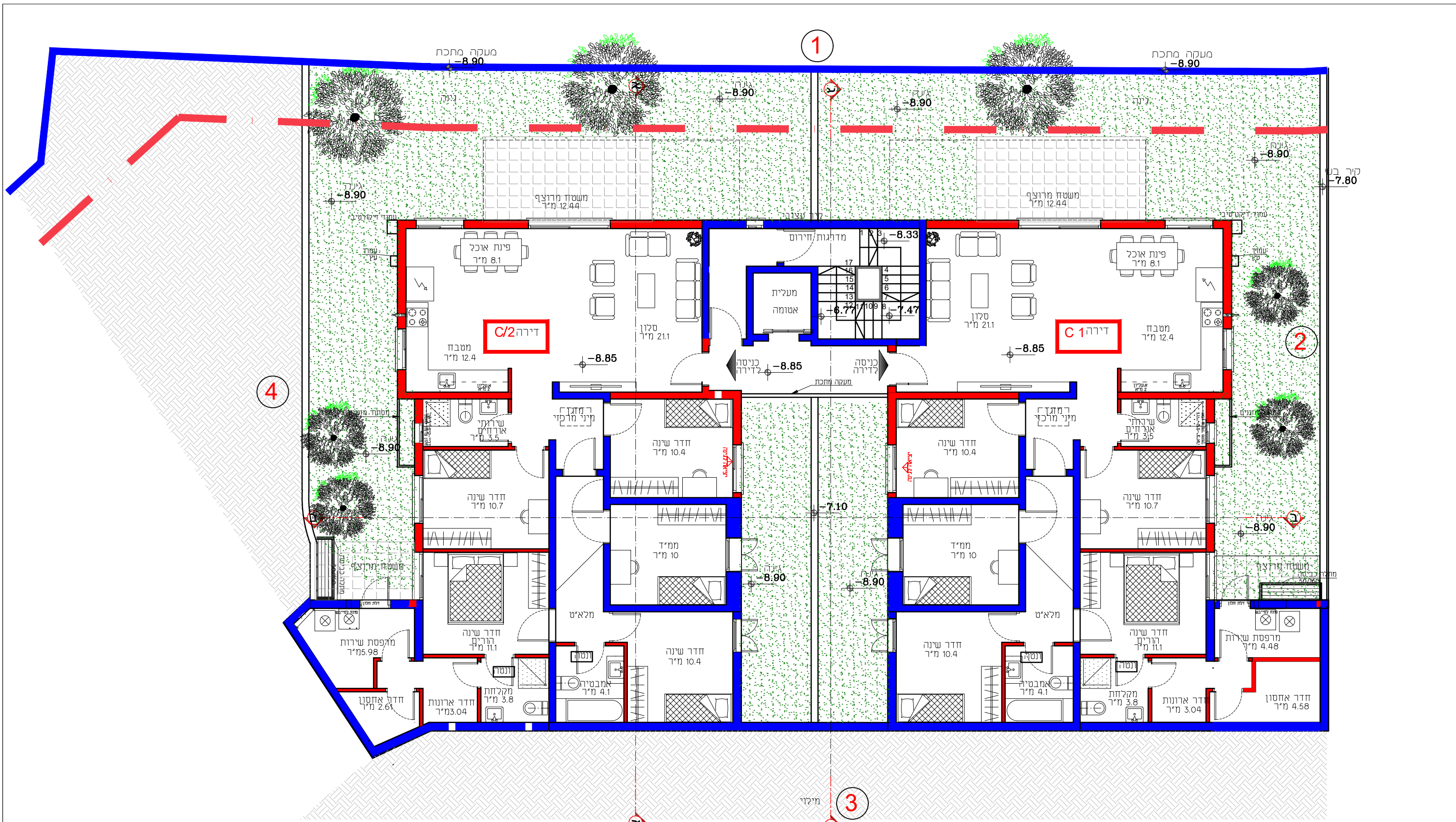
בניין C תכנית מפלס -8.85 קנ"מ 1:100
