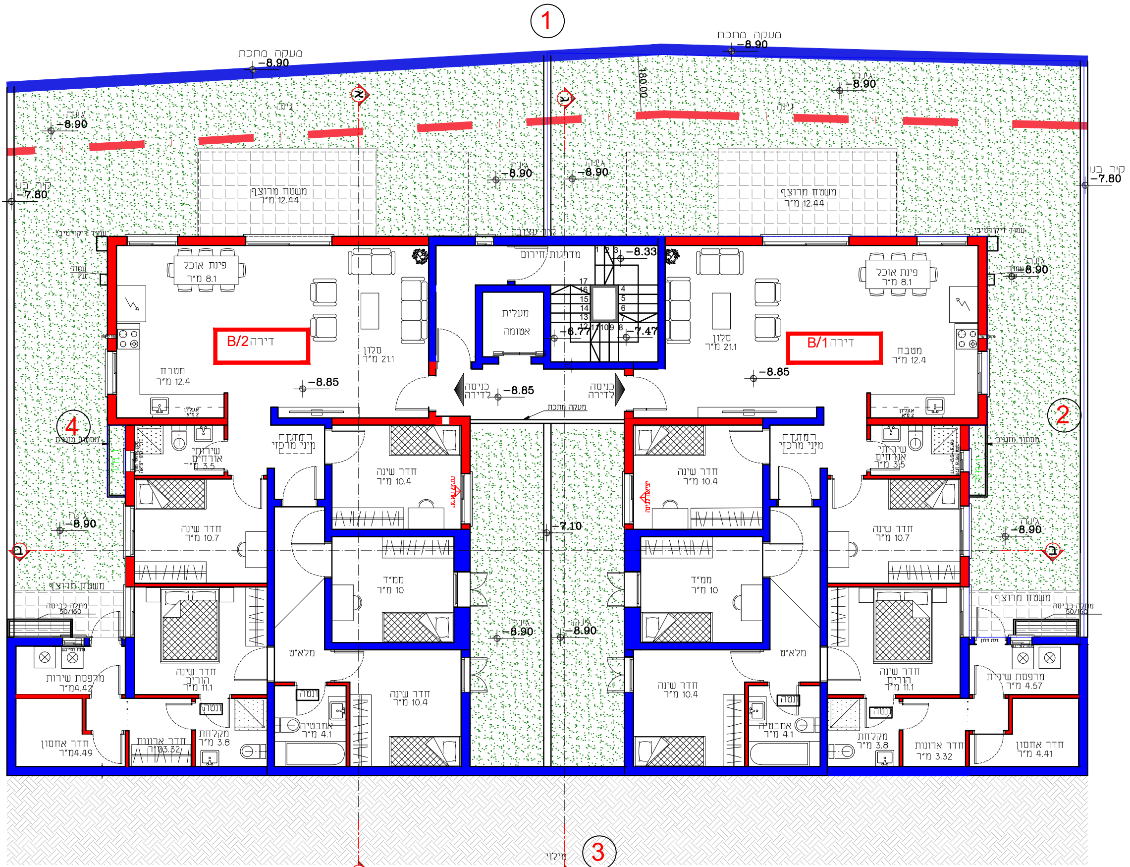
בניין B תכנית מפלס -8.85 קנ"מ 1:100
