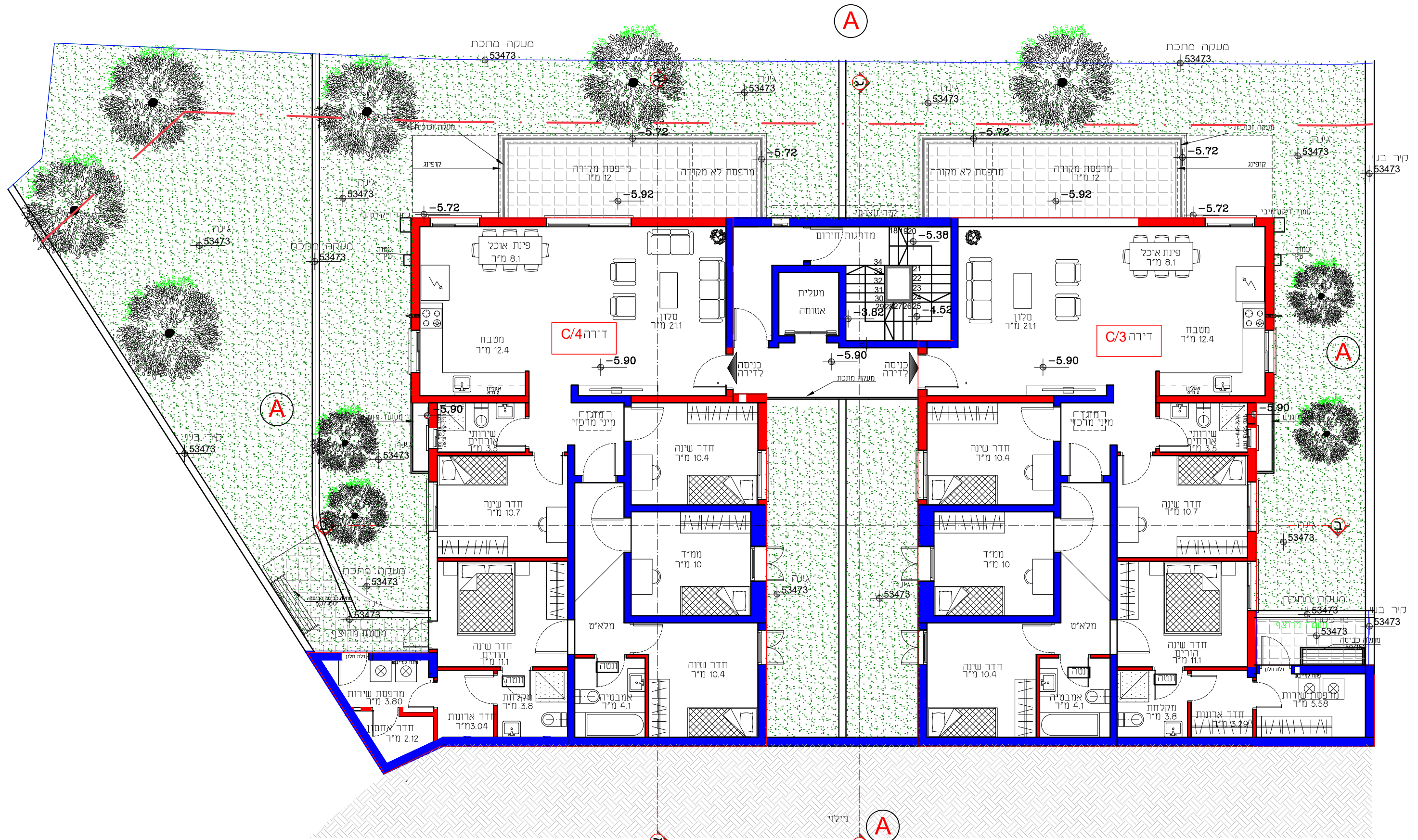
בניין C תכנית מפלס -5.90 קנ"מ 1:100
