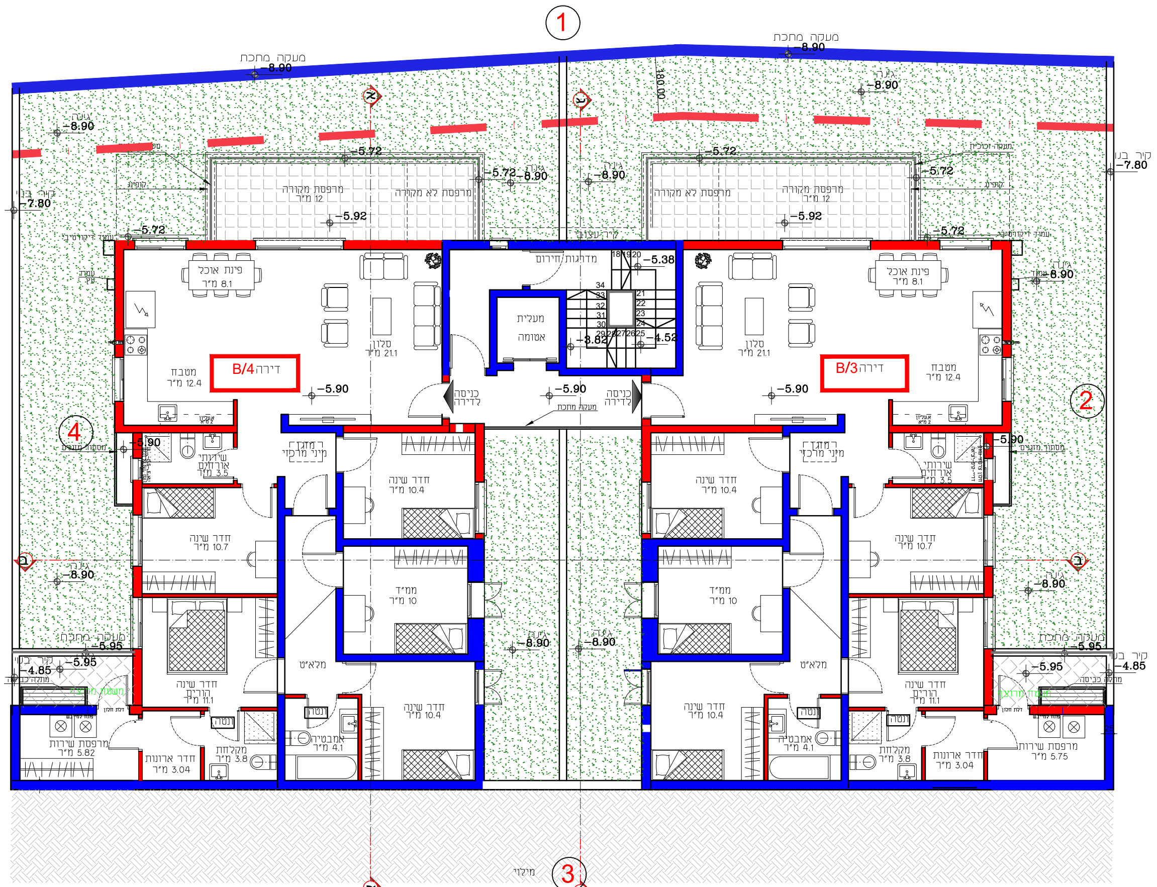
בניין B תכנית מפלס -5.90 קנ"מ 1:100
