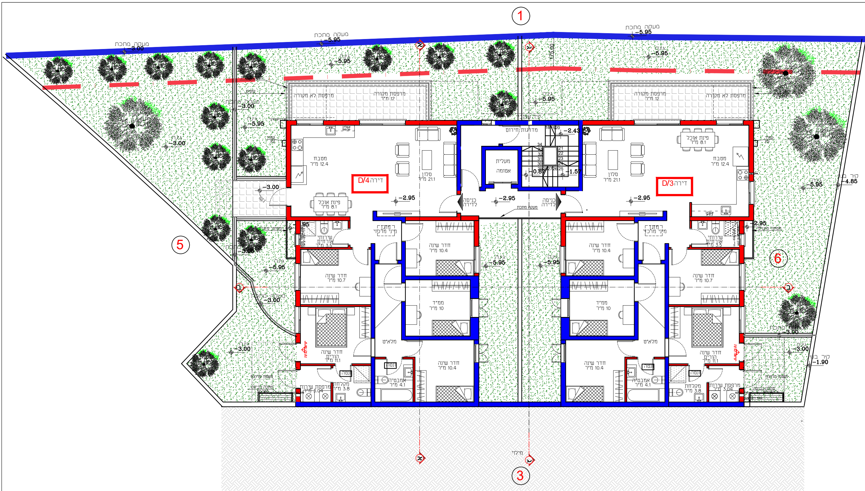
D בניין תכנית מפלס -2.95 קנ"מ 1:100
