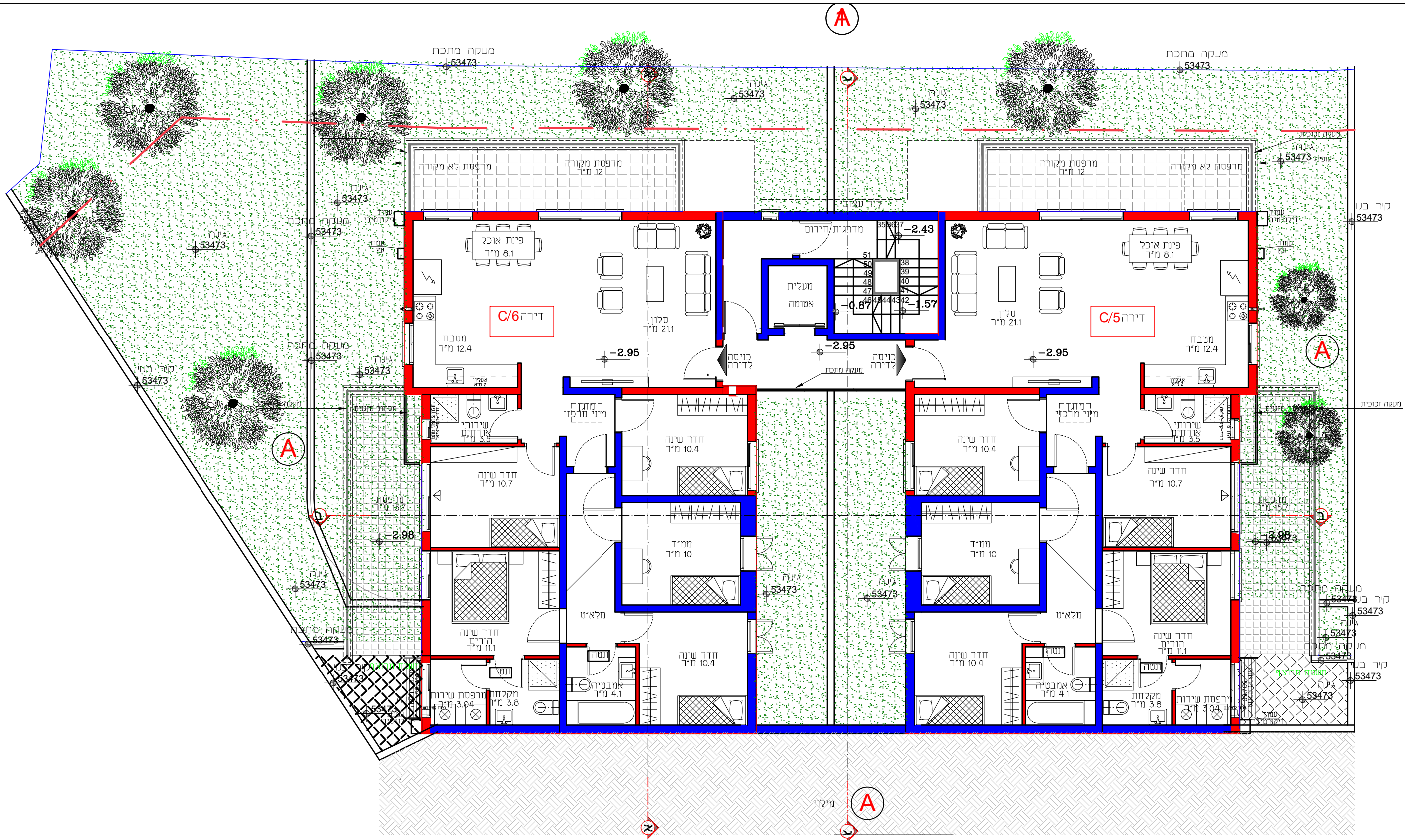
בניין C תכנית מפלס -2.95 קנ"מ 1:100
