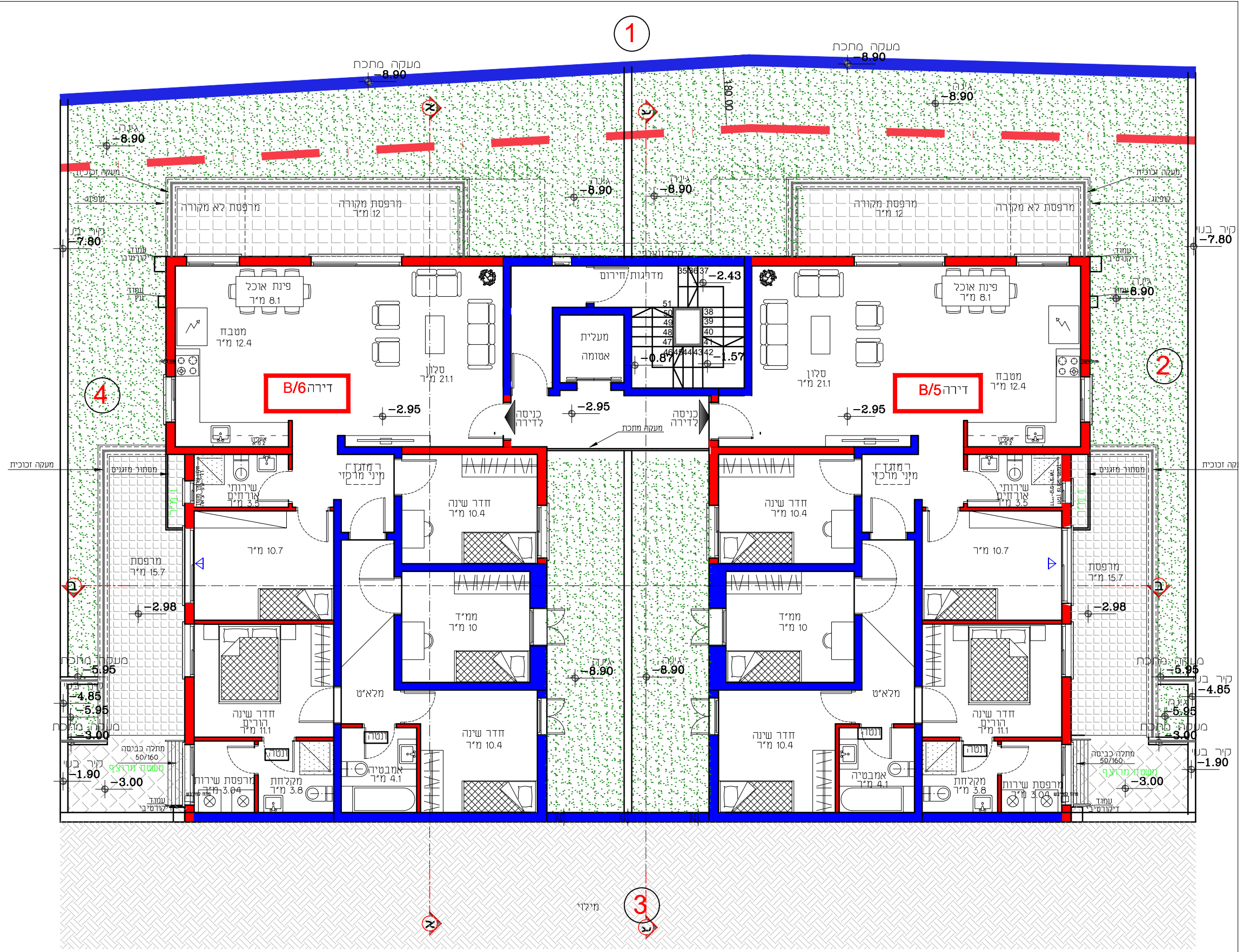
בניין B תכנית מפלס -2.95 קנ"מ 1:100
