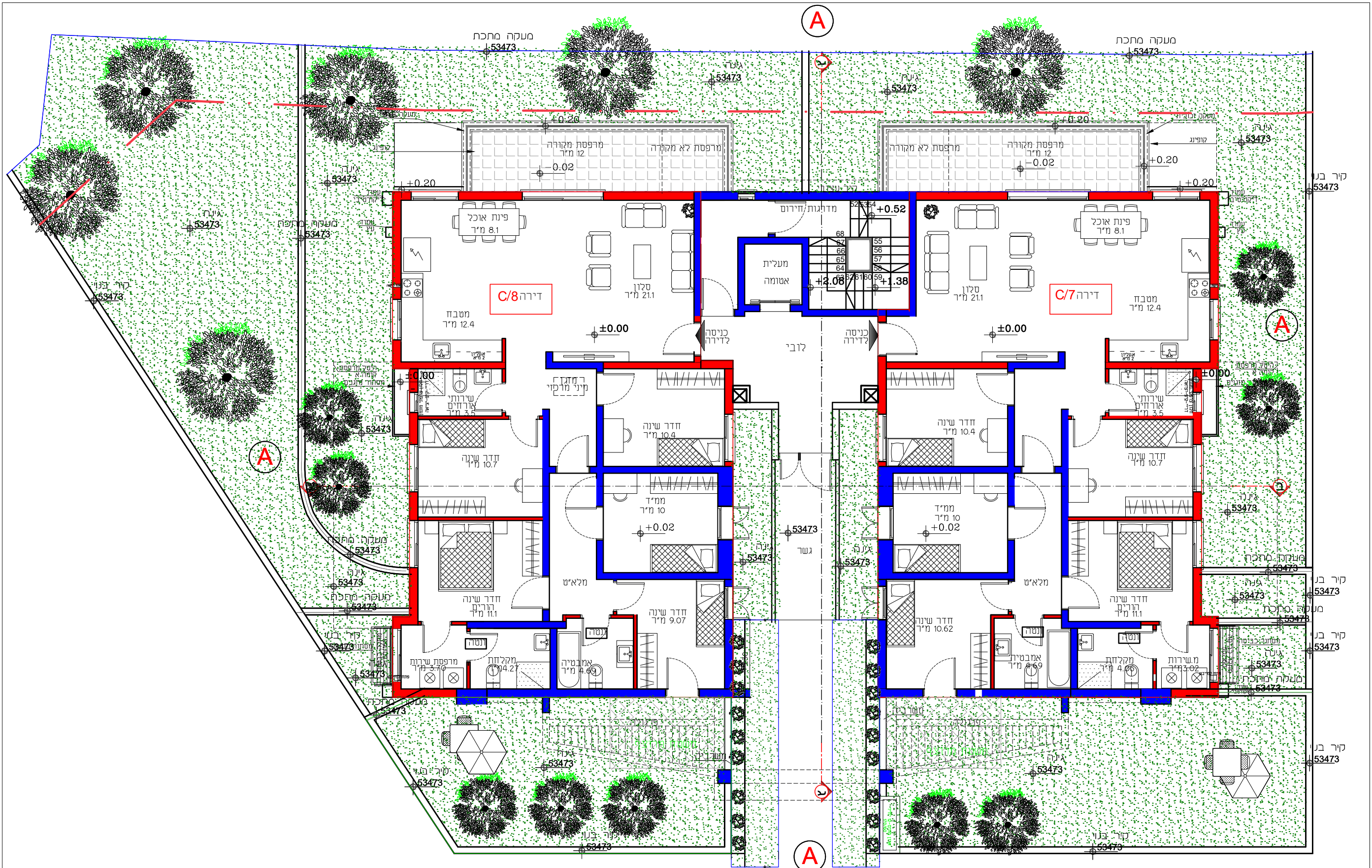
בניין C תכנית מפלס ±0.00 קנ"מ 1:100
